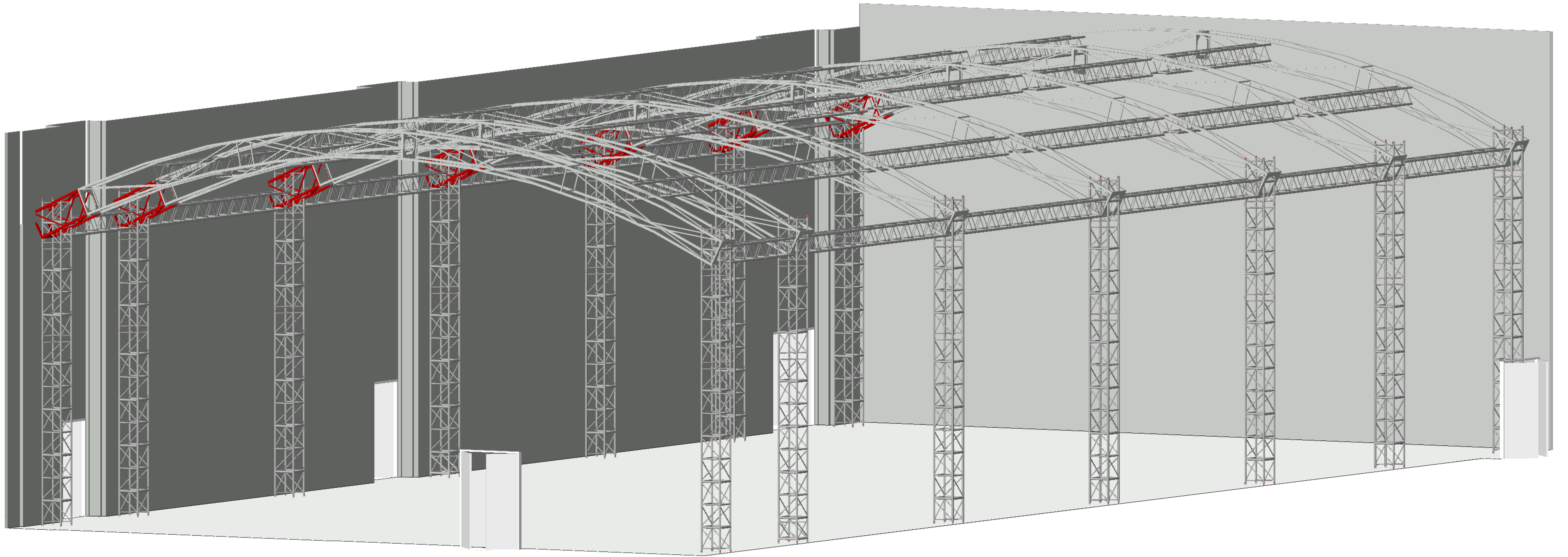
6 3D right iso Scale: 1:30
